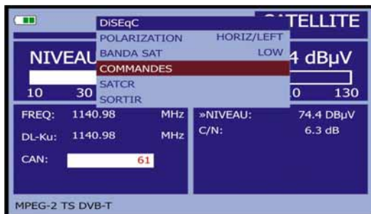
Figure 74.- Écran des commandes DiSEqC.
