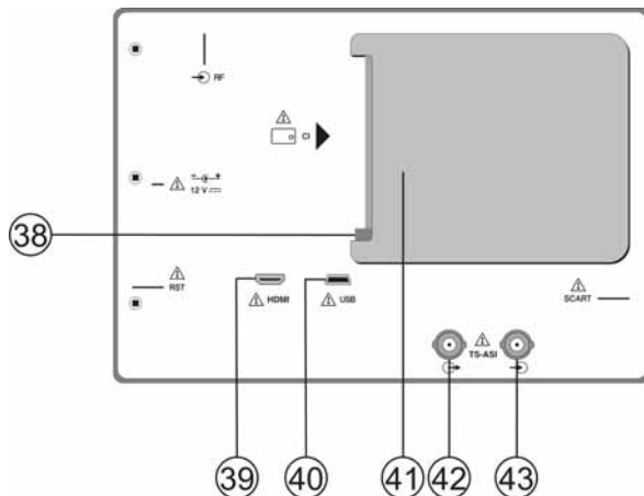
Figure 8.- Panneau postérieur.
