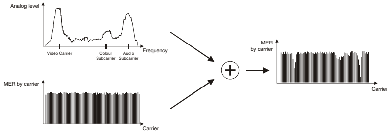
Figure 55.- Schéma d'interférence par signal TV analogique sur le canal numérique.
