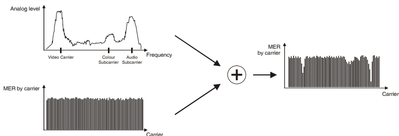
Figura 55.- Esquema de interferencia por señal TV analógica sobre canal digital.
