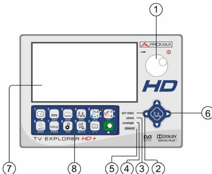
Figure 3.- Panneau frontal.
