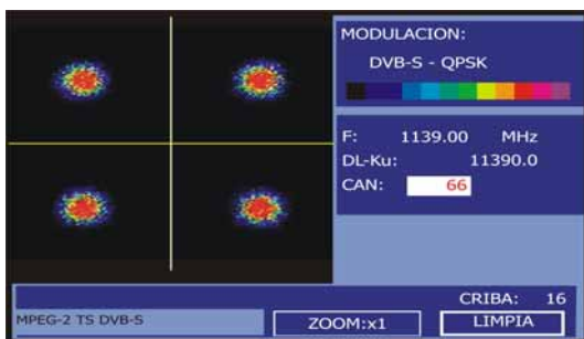
Figura 49.- Diagrama de constelación. Señal DVB-S (QPSK).
