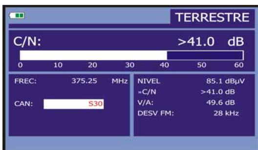
Figura 27.- Medida de la relación portadora/ruido (C/N).
