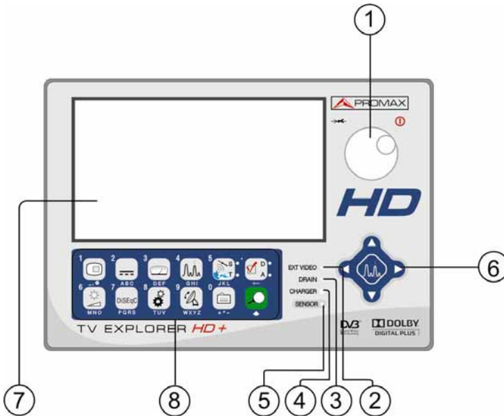
Figura 3.- Panel frontal.
