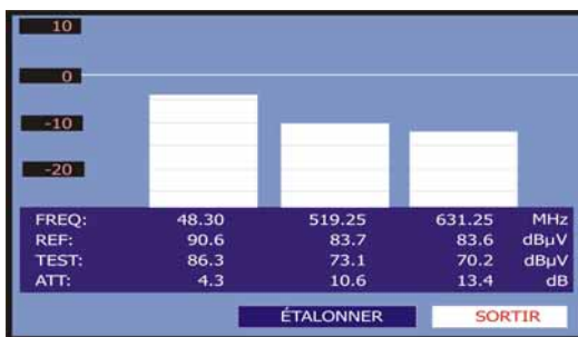
Figura 13.- Test d'Atténuation. Bande terrestre.
