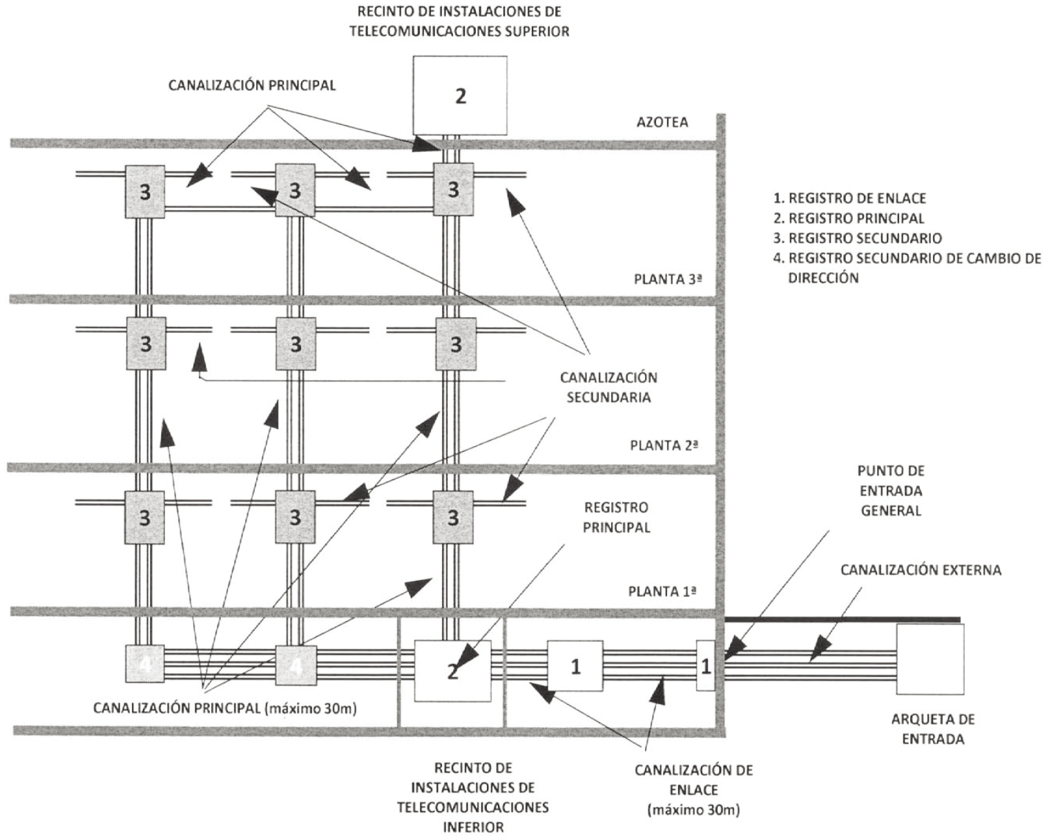
APENDICE 5: Esquema general de canalizaciones con varias verticales
