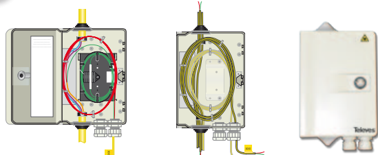
Cuando Nº PAUs > 15 Cajas de segregación
