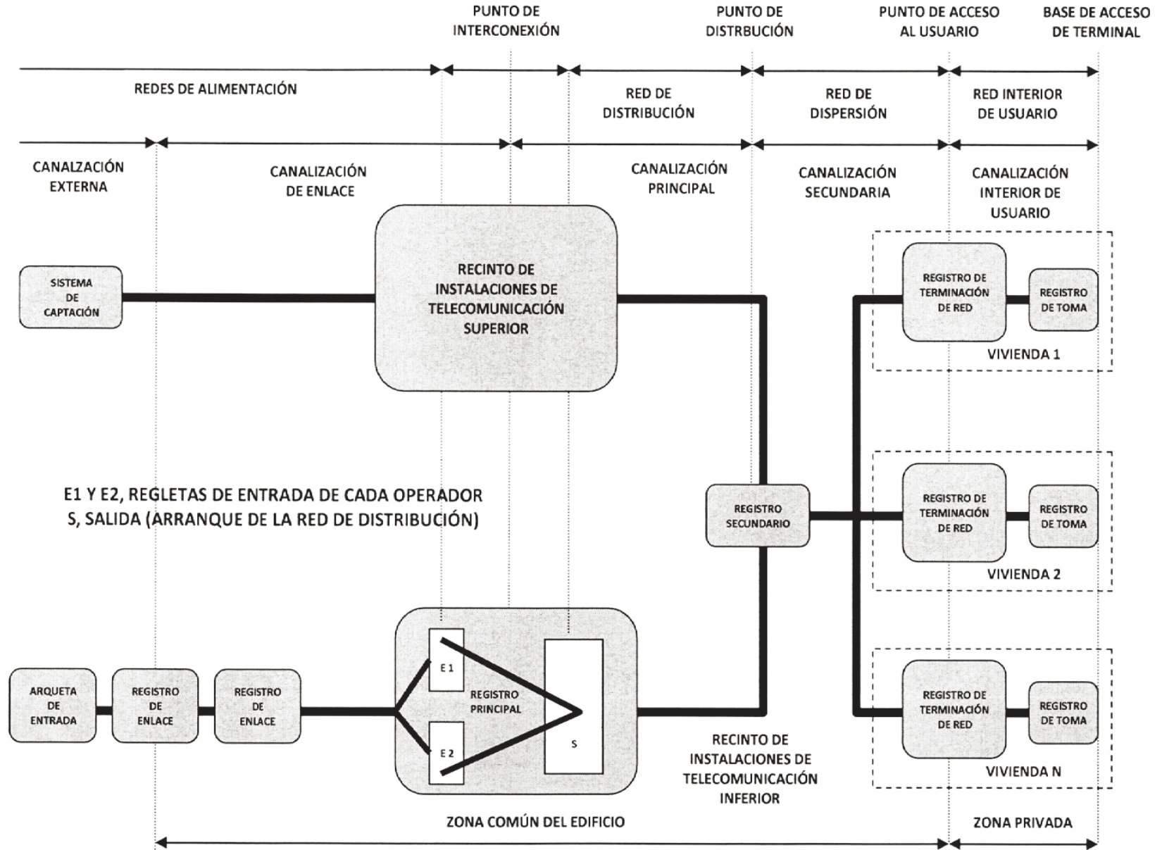
APENDICE 1: Esquema general de una ICT
