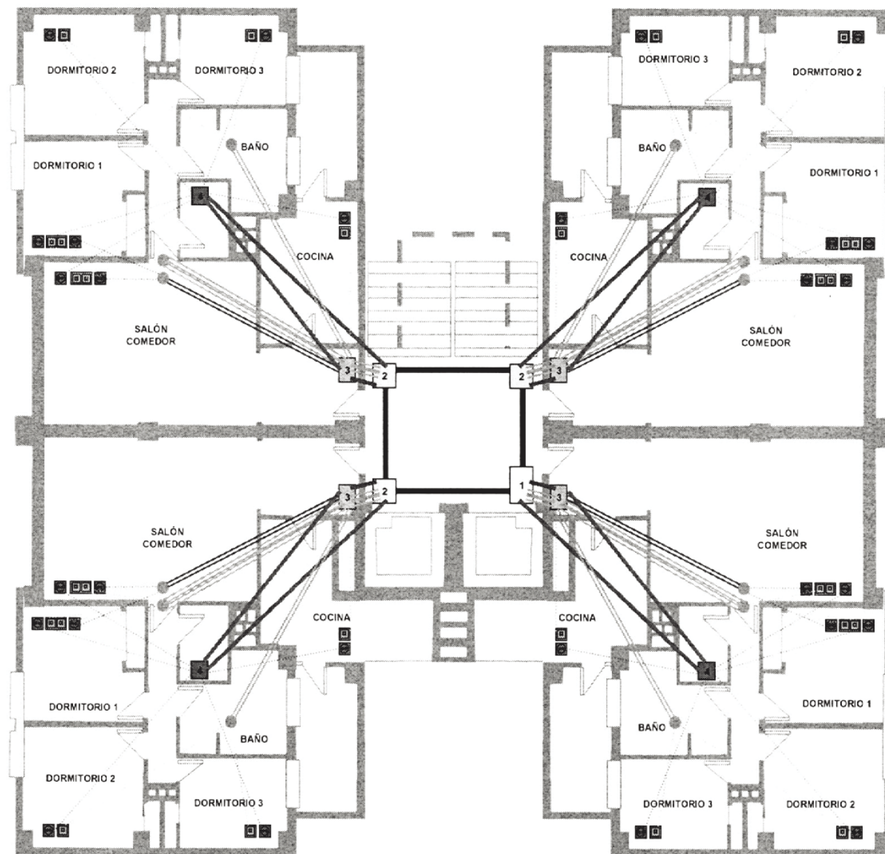
APENDICE 7: Canalización secundaria y red interior de usuario
