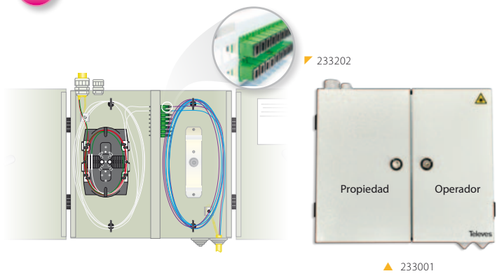
Cuando PAUs ≤ 15 Distribución en estrella desde el Registro principal del RITI
